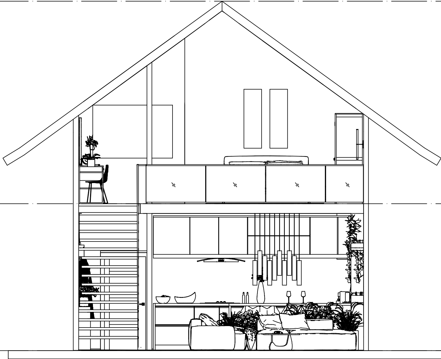
ELEVATION I-I
