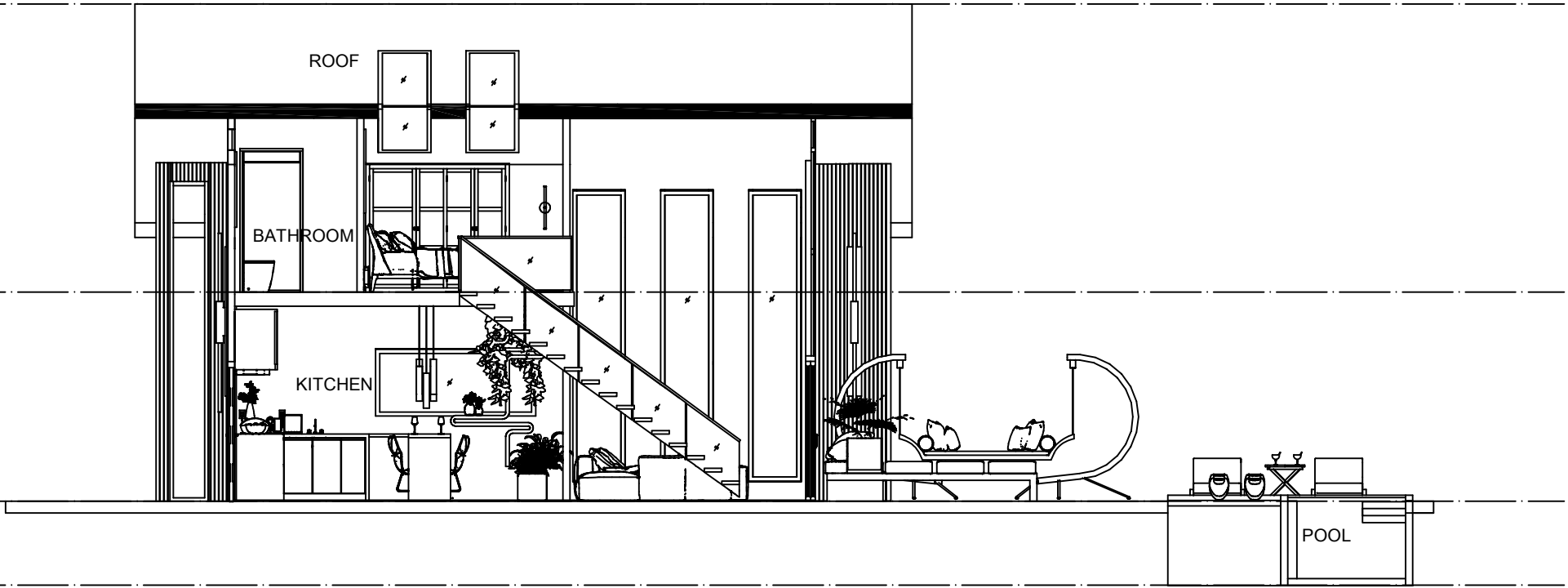
ELEVATION II-II
